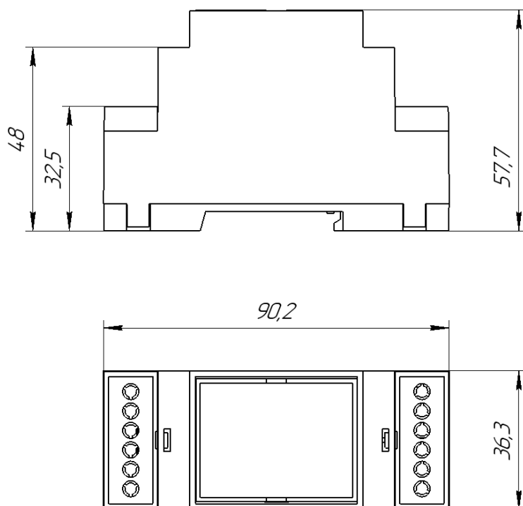
Рис. 1. Внешние размеры УЗИП RS232 (Исполнение 1).
